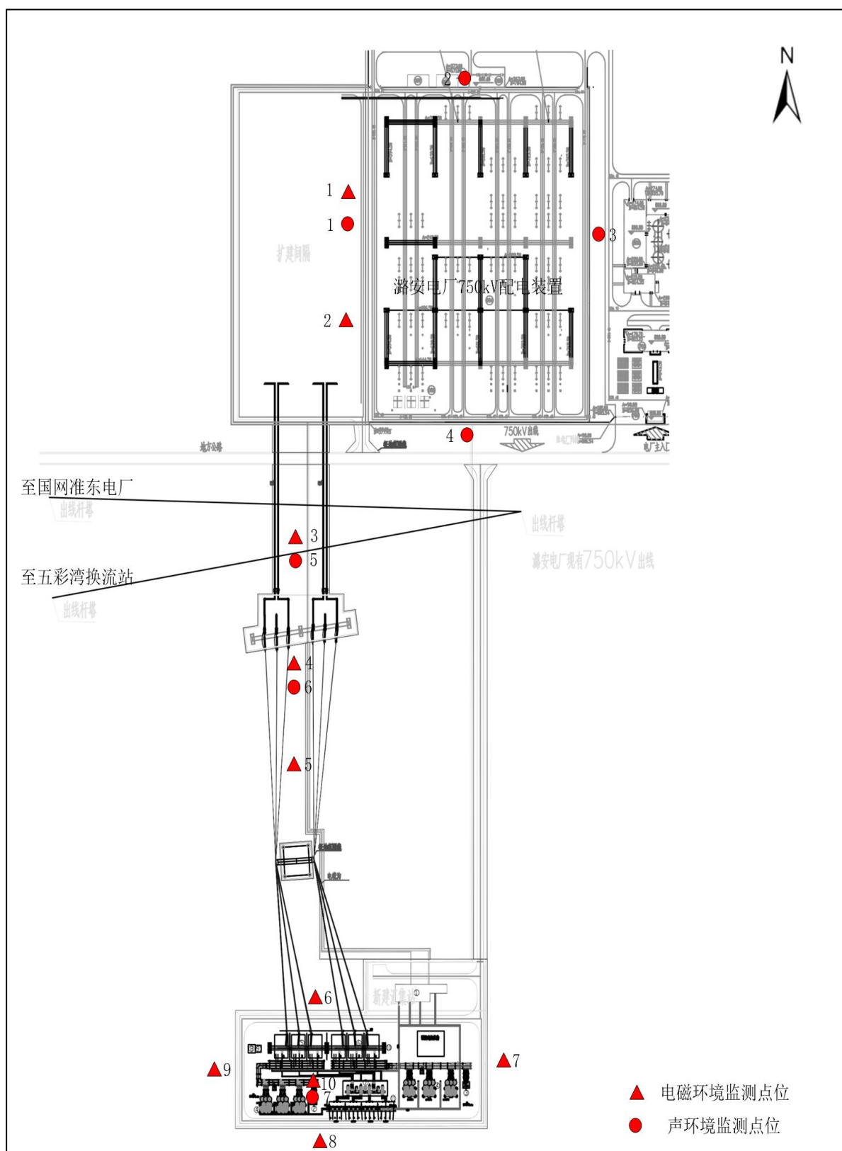
图 4-1 工频电磁场及噪声现状监测分布图
