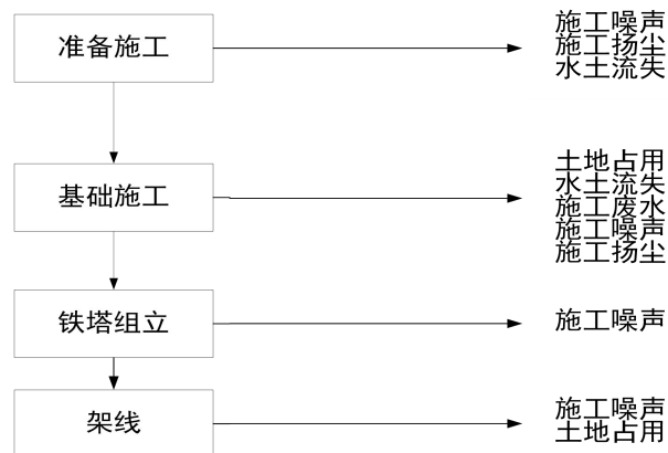
图 3-2 输电线路施工工艺及产污环节
